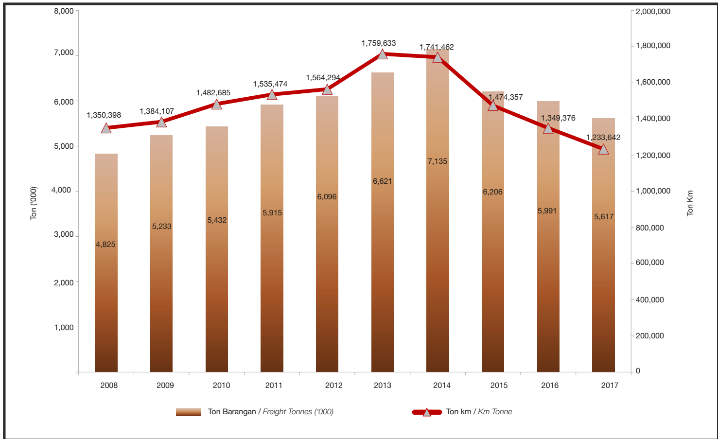
CARTA 2.3: TRAFIK BARANGAN BAGI PERKHIDMATAN KERETA TAPI TANAH MELAYU BERHAD (KTMB), 2008-2017
